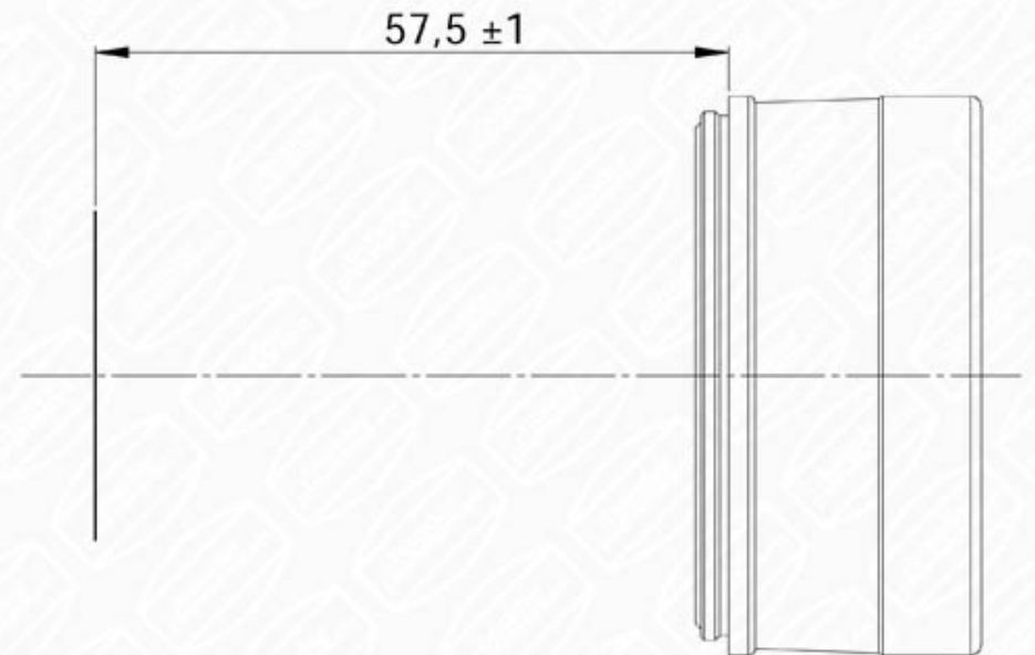
M42 (T-2)取付けリングと2インチストッパーリングを取り外したM48取付け面からのバックフォーカス
