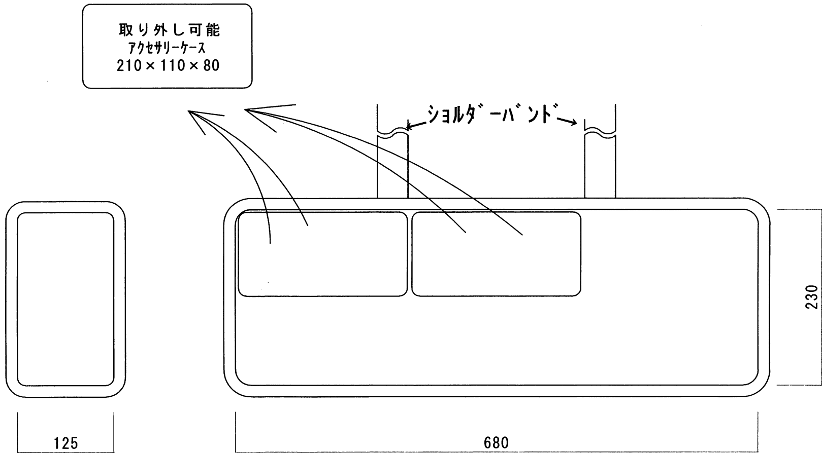
BAG202内寸図
